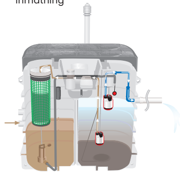
4. Utpumpning av renat vatten och behandling av överskottsslam
